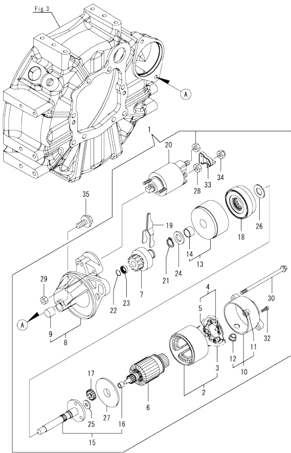
OCD50-M00530 3TNM74F-NGGE Fig.14. STARTER MOTOR
