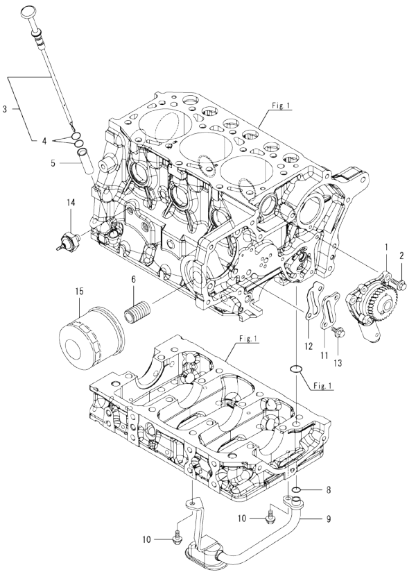
OCD50-M00530 3TNM74F-NGGE Fig.8. LUB. OIL SYSTEM
