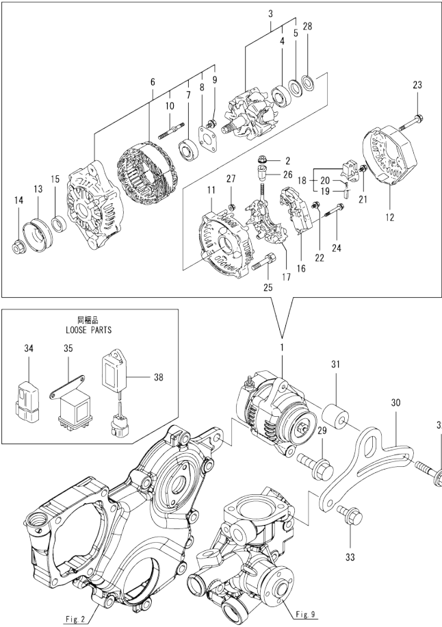
Fig.15. GENERATOR
